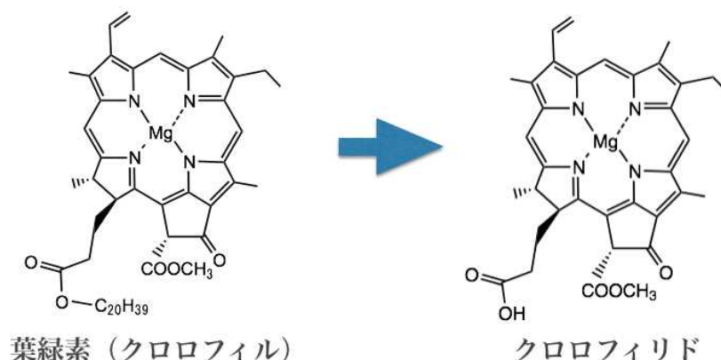
図1 葉緑素（クロロフィル）とクロロフィリドの構造
